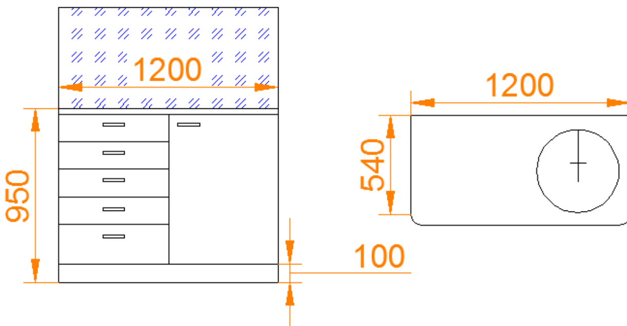
Skice Nr.3 - Lete ar izlietni, 206.kabinetā
