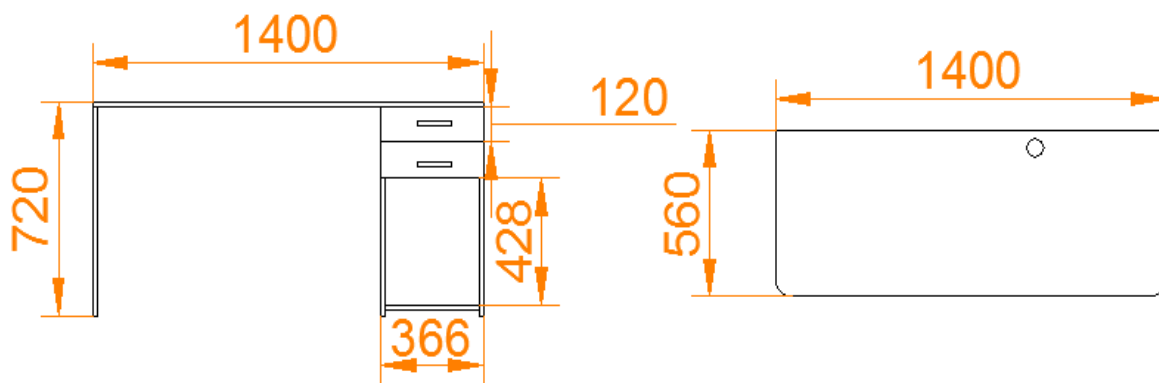
Skice Nr.1 - Datorgalds 204. un 206.kabinetā
