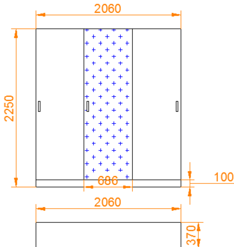
Skice Nr.5 - Lielais skapis 204.kabinetā
