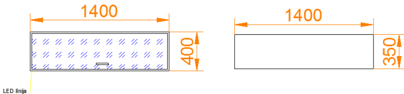
Skice Nr.2 - Skapītis virs datorgalda un virs izlietnes skapīti 206.kabinetā
