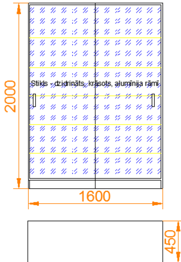
Skice Nr.3 – Materiālu skapis zobārstniecības kabinetā
