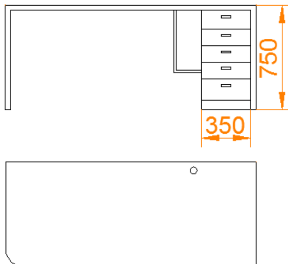
Skice Nr.8 – Datorgalds virsmāšas kabinetā
