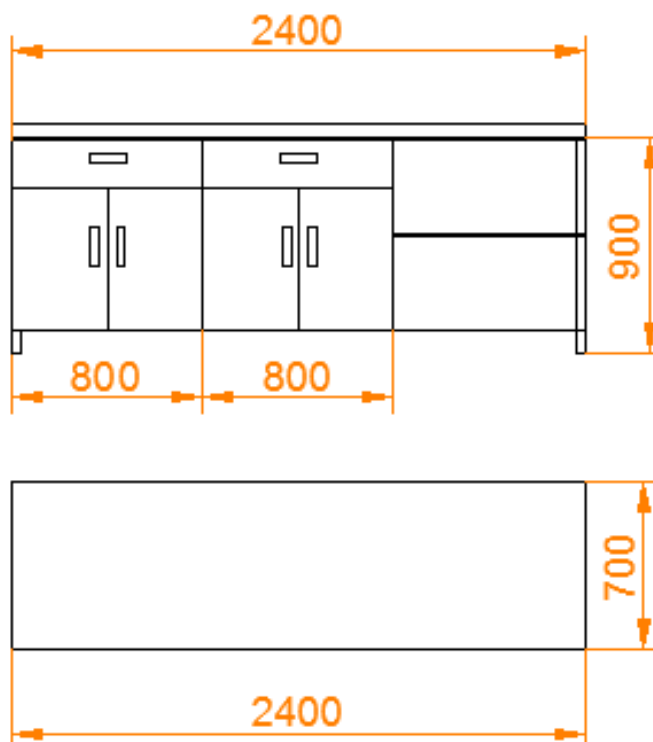
Skice Nr.26 – Nerūsējoša tērauda darbagalds ar atvilknēm, durtiņām un plauktiem
