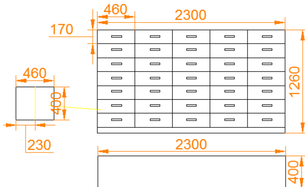
Skice Nr.23 – Reģistratūras skapis kartiņām – lielais
