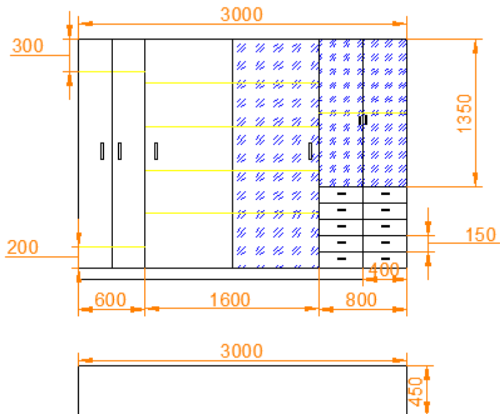
Skice Nr.10 – Materiālu skapis ar durvīm un atvilknēm virsmāskabinētā
