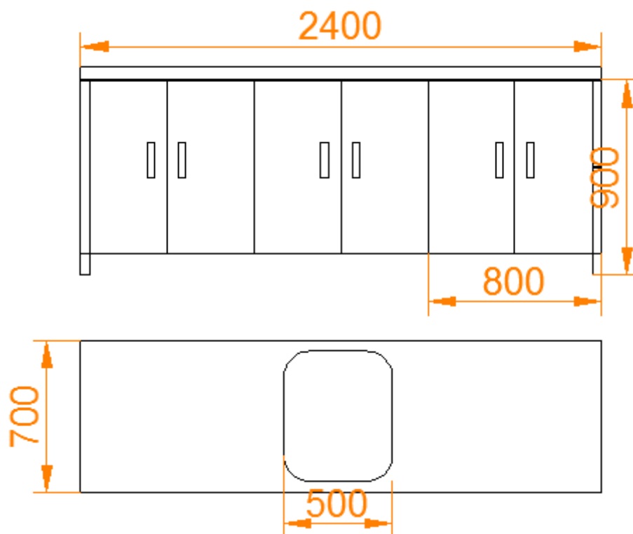
Skice Nr.26 – Nerūsējoša tērauda darbagalds ar atvilknēm, durtiņām un plauktiem
