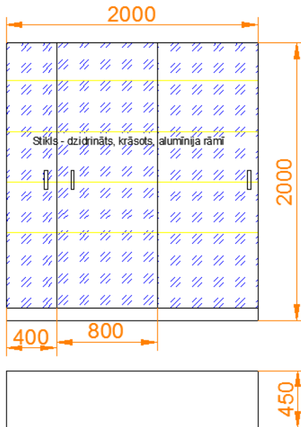
Skice Nr.4 – Dokumentu un materiālu skapis kabinetā Nr.18
