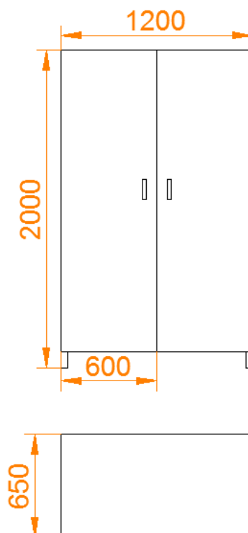
Skice Nr.28 – Nerūsējoša tērauda divvārtņu skapis
