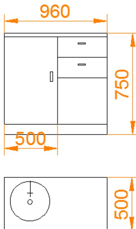
Skice Nr.6 – Izlietnes skapis ar atvilknēm rentģentelpā
