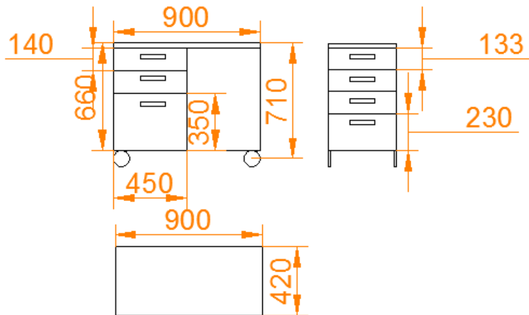
Skice Nr.21 - Skapis uz riteņiem un divpusējām atvilkņēm bērnu nodaļā
