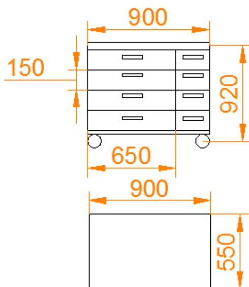
Skice Nr.36 – Medicīnas skapis uz riteņiem ar atvilkņēm
