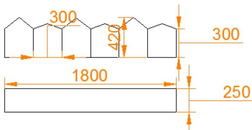
Skice Nr.22 – Sienas plaukts bērnu stūrim
